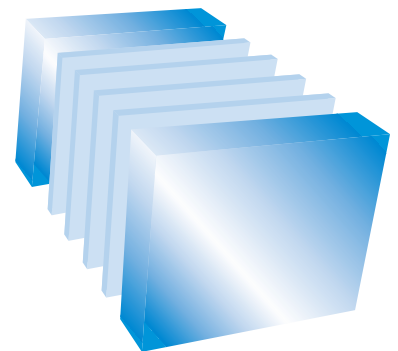
SP410 (oude benaming 44.4) bestaat uit 2 glasplaten van 4 mm waartussen zich 4 PVB-filmen bevinden, elk 0,38 mm dik.
