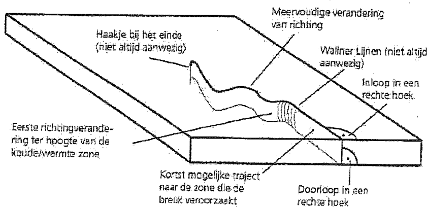
Afbeelding 1: Kenmerkend beeld van een thermische breuk
